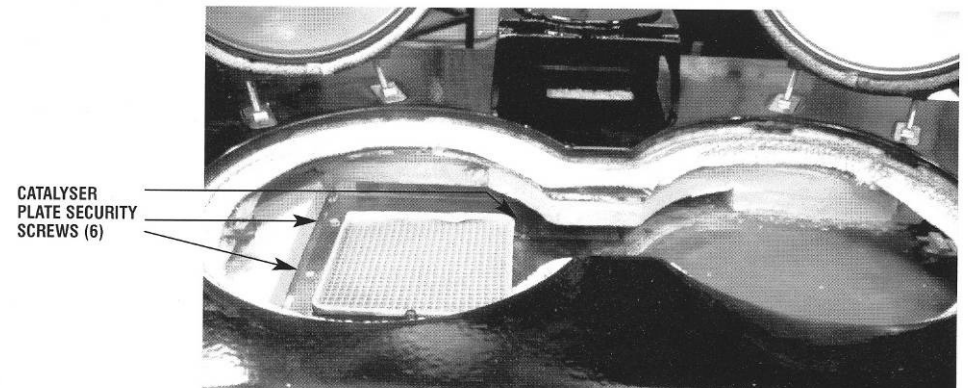
Fig. 8 - Catalyser
